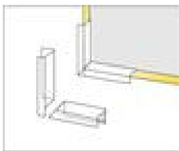
Przycięcie profilu ceowego przy narożniku wewnętrznym
